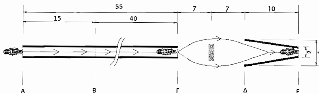
ΣΧΕΔΙΟ 1 ΑΠΕΙΚΟΝΙΣΗ ΧΩΡΟΥ ΔΟΚΙΜΑΣΙΑΣ ΚΙΝΗΣΗΣ ΜΕ ΑΠΟΦΥΓΗ ΕΜΠΟΔΙΟΥ
